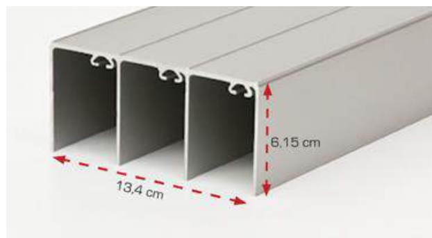
Dreiläufige Führungsschiene
