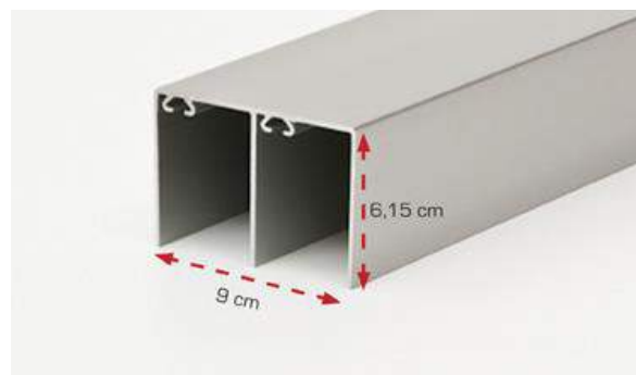
Zweiläufige Führungsschiene
